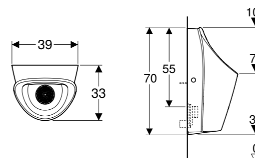
Geberit Selnova L
